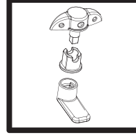
C Kapak Kilit Takımı X 2 Adet Cover Lock Set X 2 Pieces
